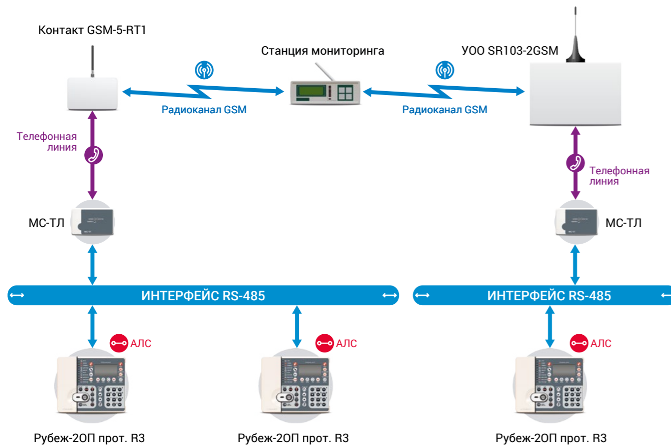
Схема организации системы мониторинга по каналу GSM
