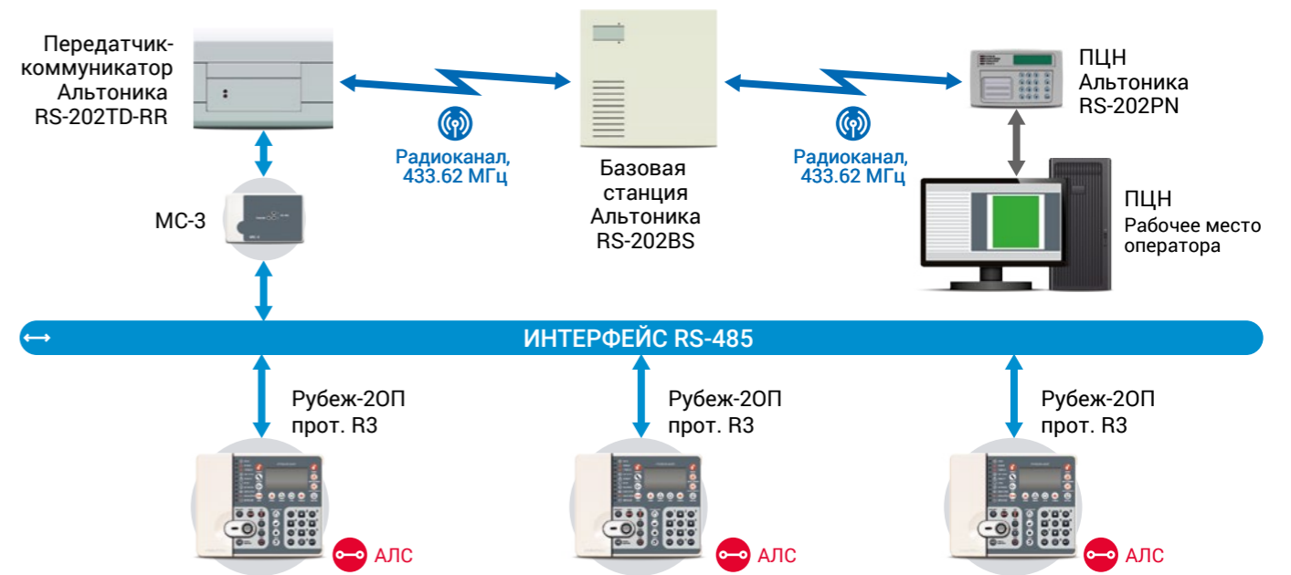
Схема передачи извещений от приборов интерфейса RS-485 на мониторинговые станции по радиоканалу
