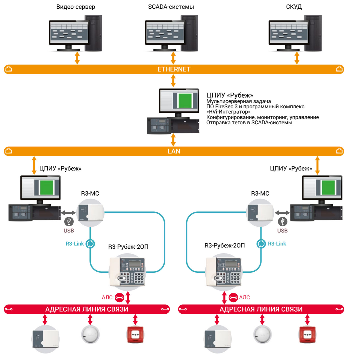
Схема реализации ЦПИУ «Рубеж»
