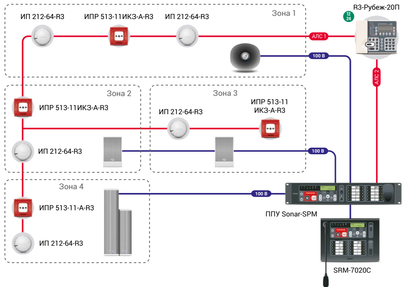
Схема систем оповещения и управления эвакуацией с использованием моноблока Sonar-SPM
