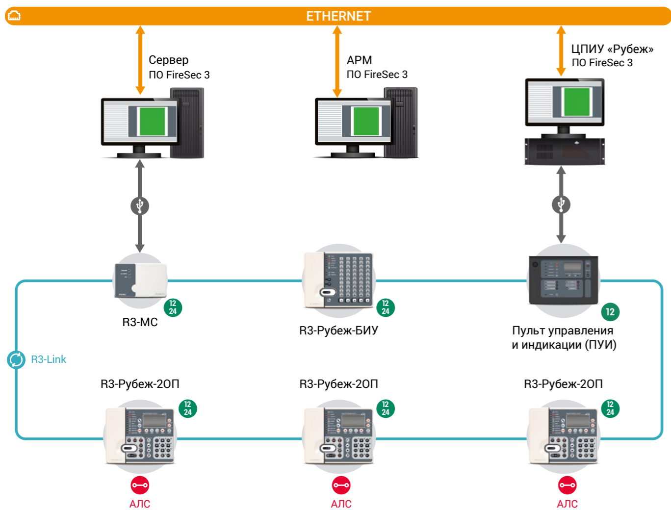
Схема организации связи интерфейса R3-Link с компьютером
