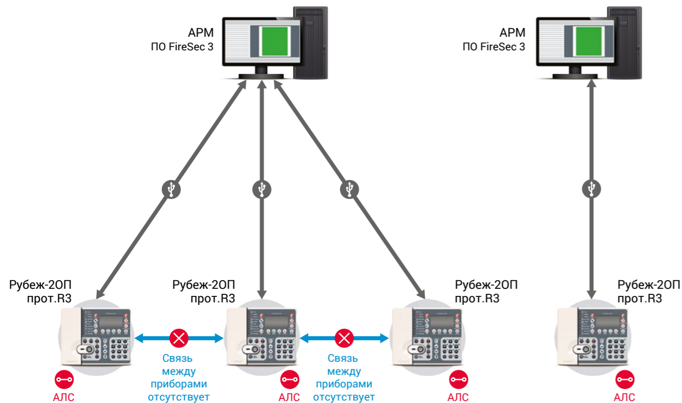
Схема подключения приборов «Рубеж-20П» прот. R3 к компьютеру по USB
