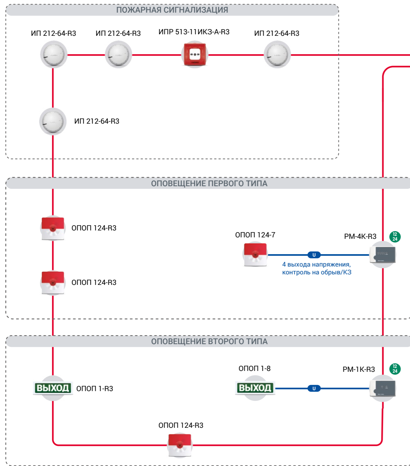
Схема систем оповещения и управления эвакуацией
