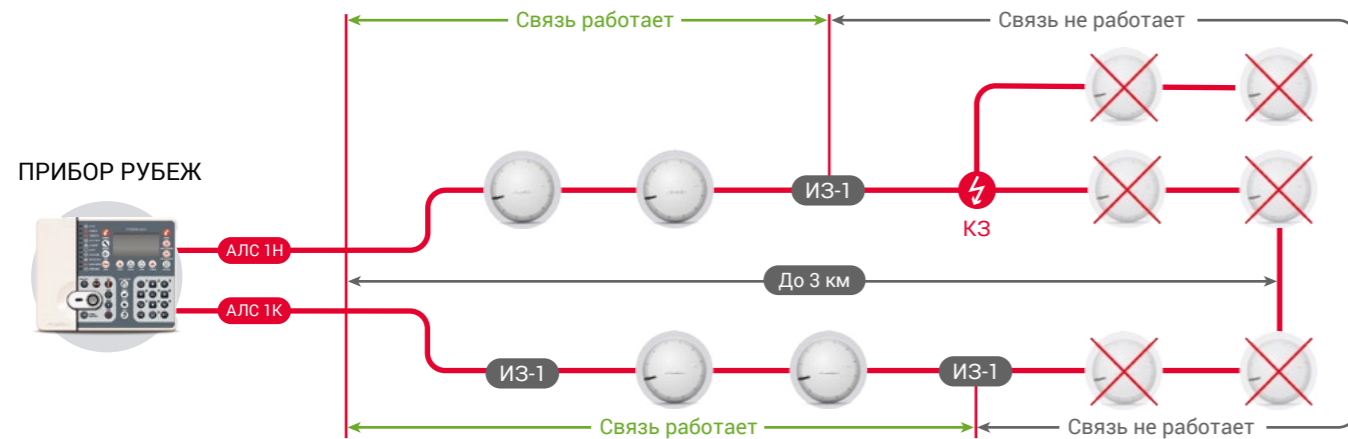
Схема кольцевой топологии адресных линий связи при коротком замыкании
