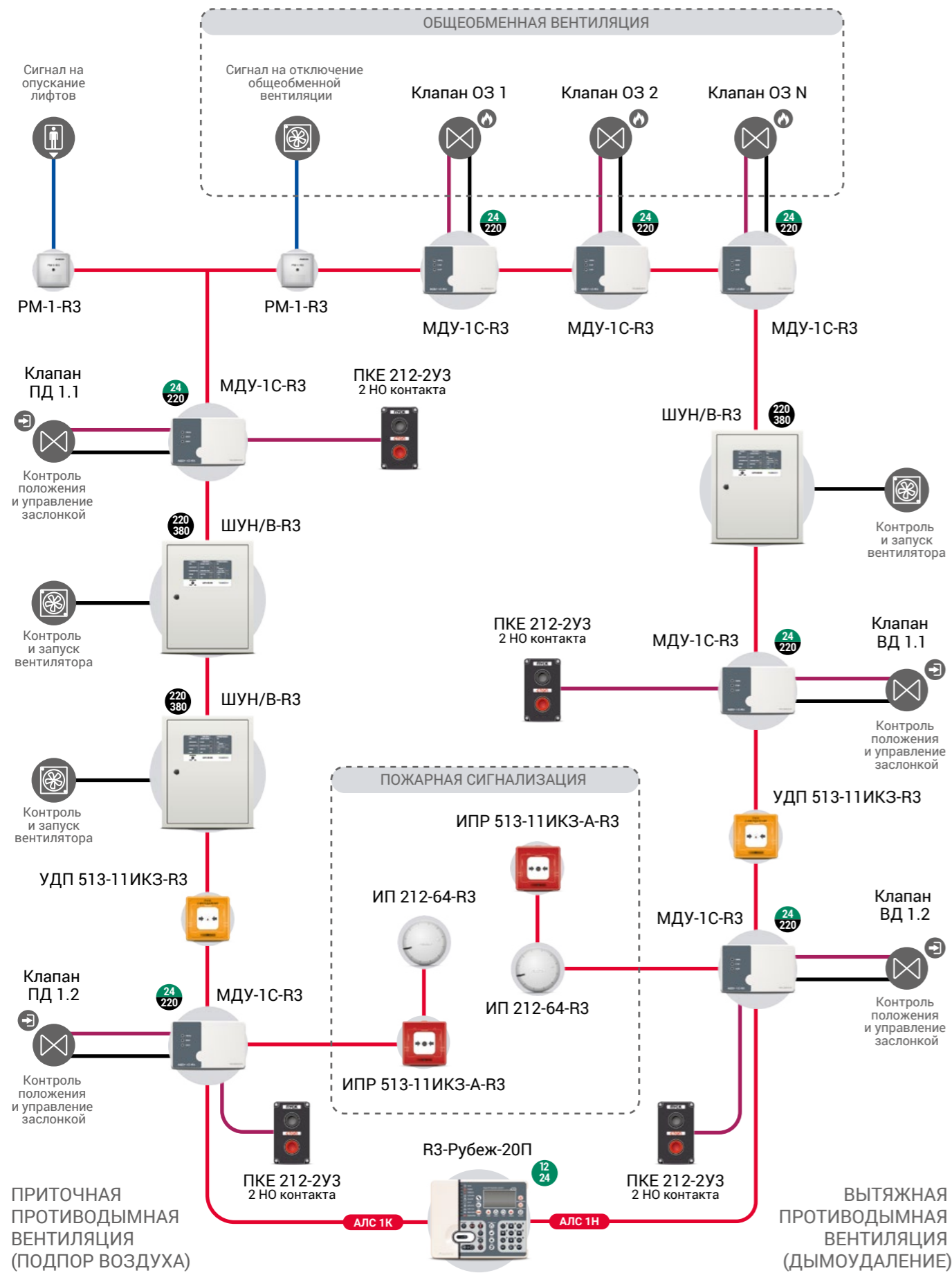
Схема систем управления противодымной вентиляцией
