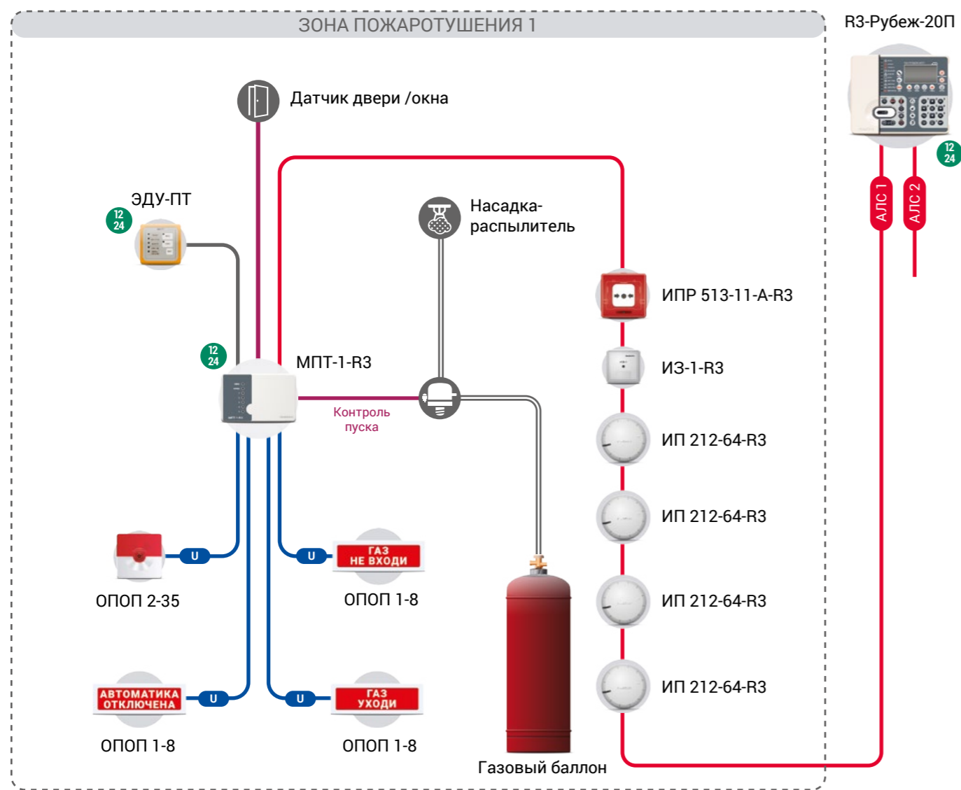
Схема системы управления газовым пожаротушением
