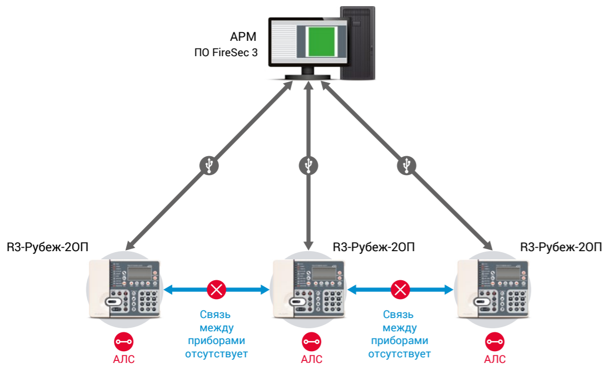
Схема подключения приборов «R3-Рубеж- 20П» к компьютеру по USB
