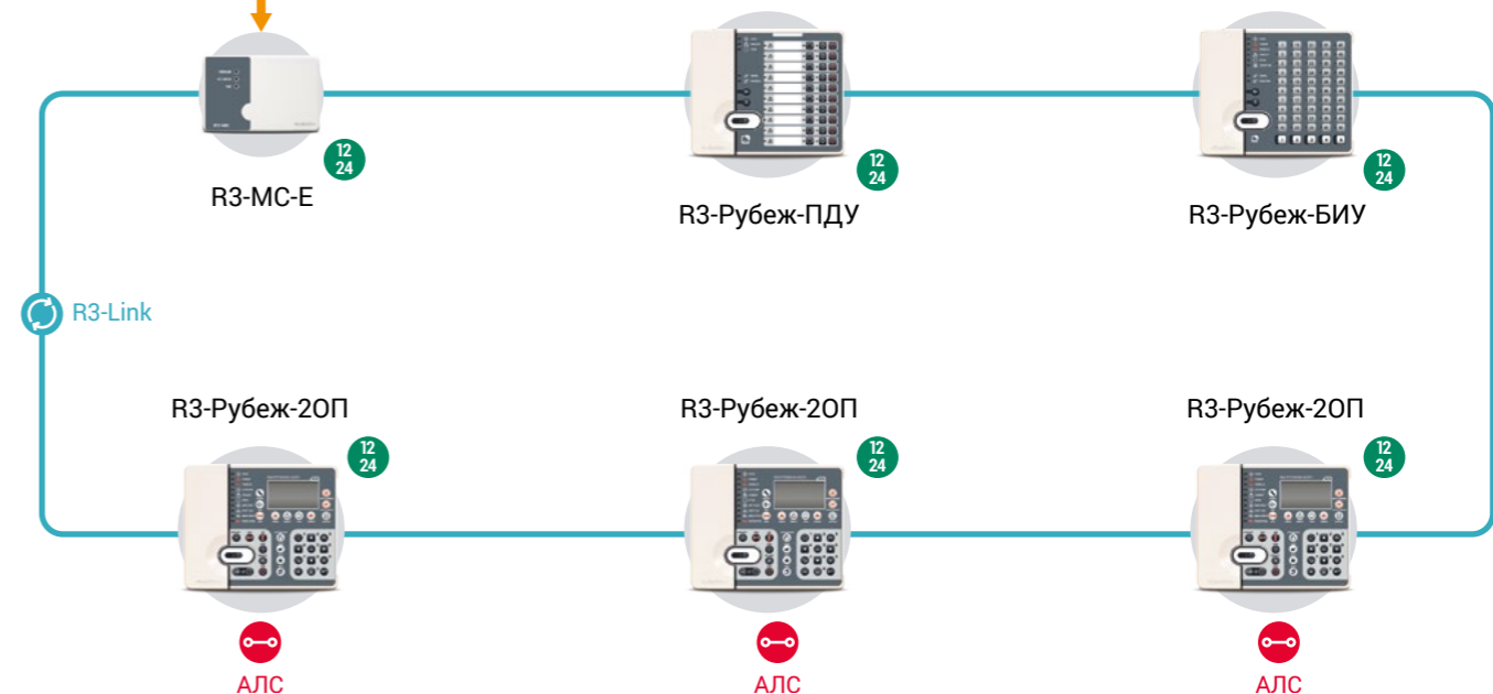
Схема организации связи двух разных интерфейсов R3-Link с компьютером
