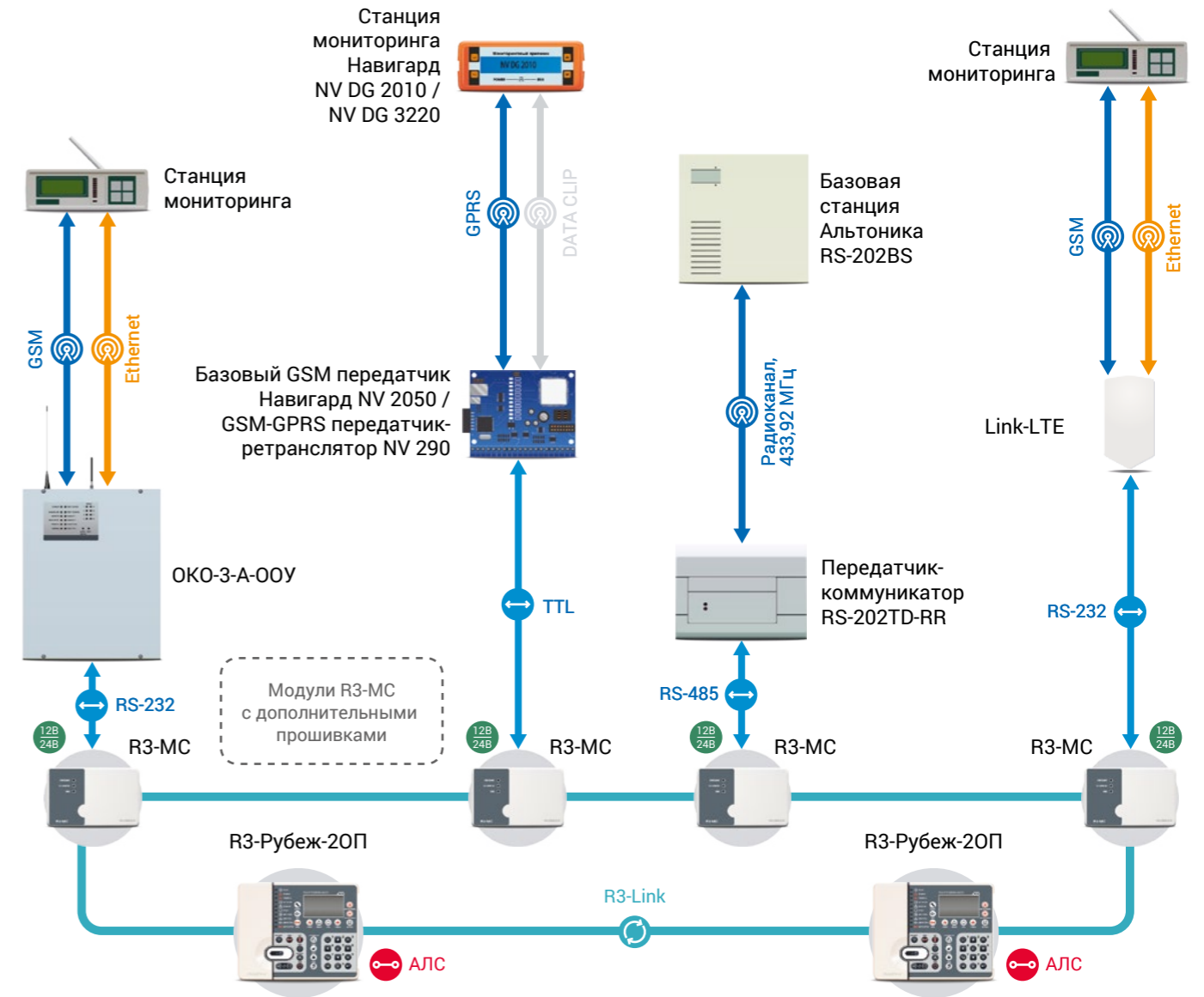
Схема передачи тревожных сообщений от приборов интерфейса R3-Link на мониторинговые станции
