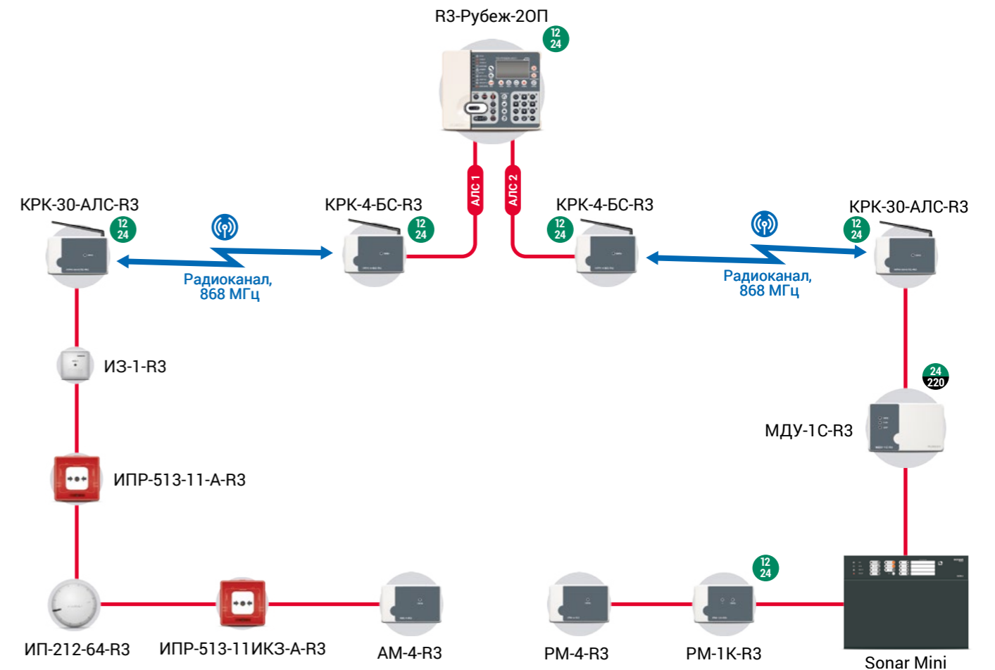
Схема радиоканального удлинения АЛС
