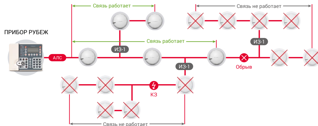
Схема работоспособности радиальной с ответвлениями топологии адресных линий связи
