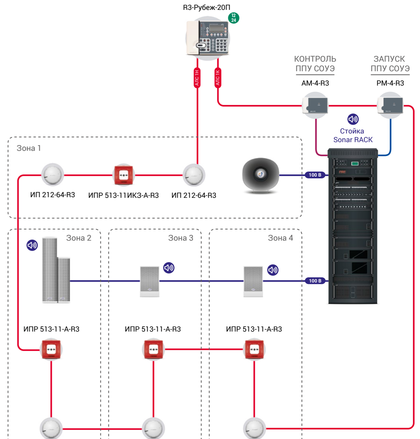
Схема систем оповещения и управления эвакуацией на базе стоечного оборудования Sonar
