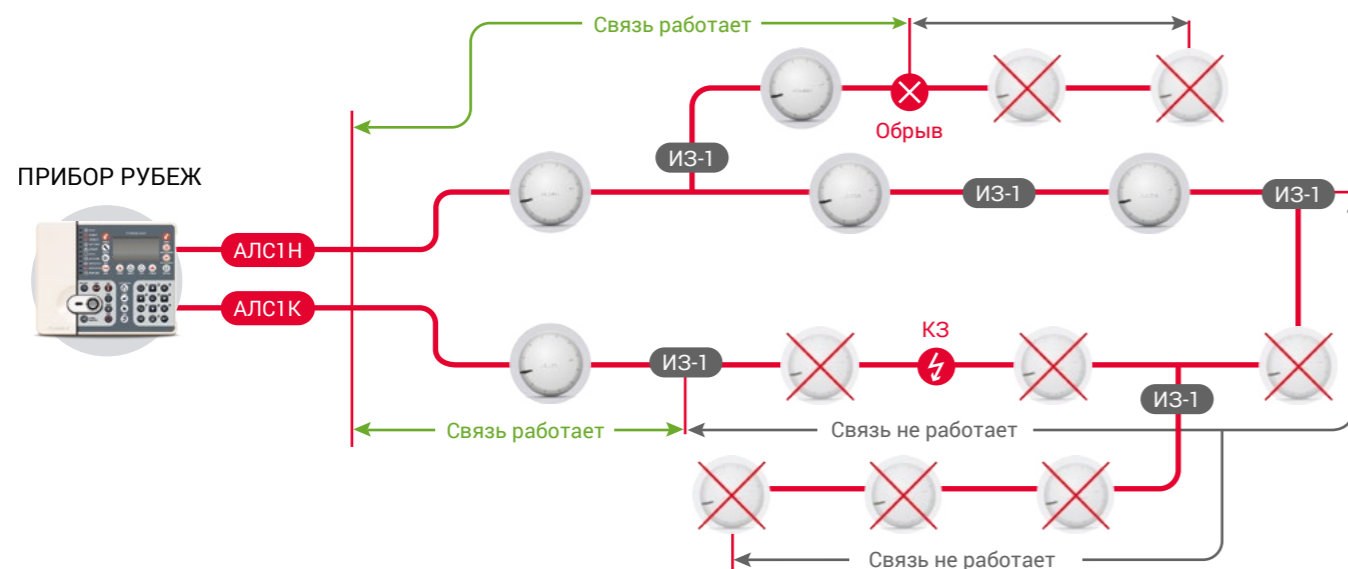
Схема кольцевой с ответвлениями топологии адресных линий связи
