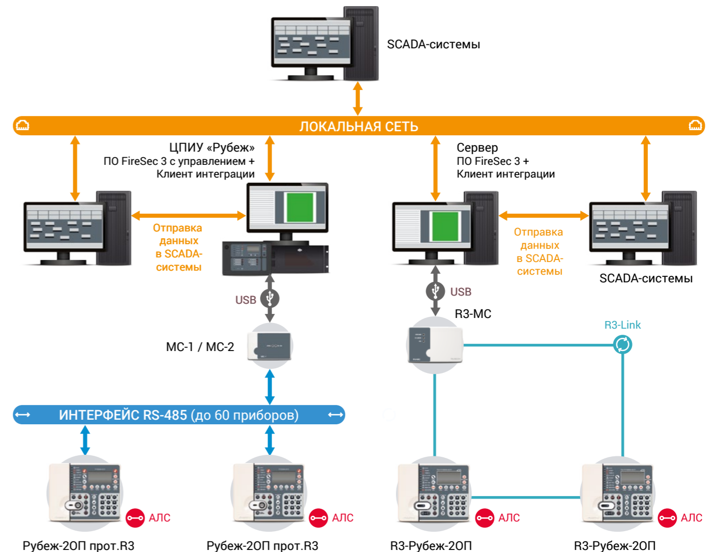
Схема реализации ПО «Клиент интеграции»
