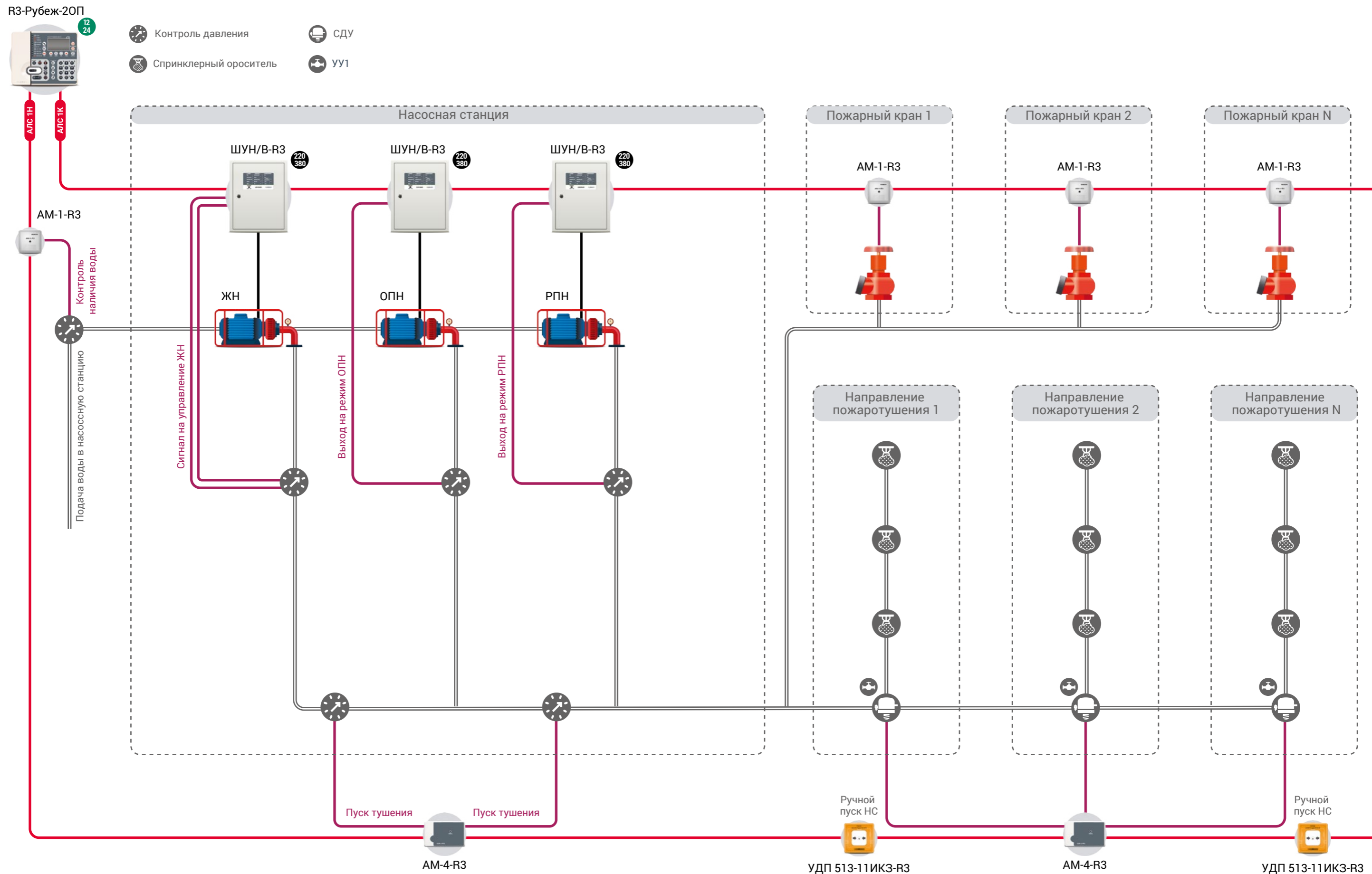
Схема организации системы управления спринклерным водяным пожаротушением
