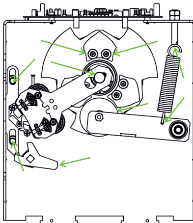
Рисунок 10.1 - Места смазки механизма
