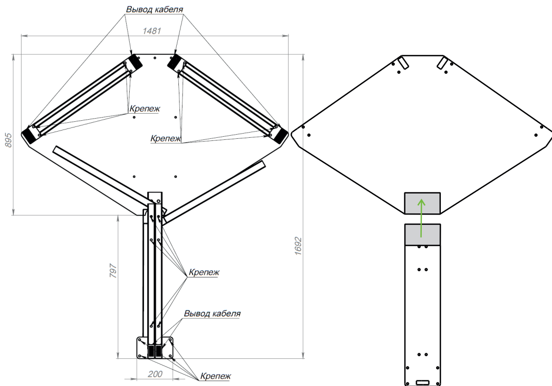
Рисунок 9.1 - Размещений крепёжных отверстий и мест вывода кабеля (слева) и трафарет (шаблон) турникета (справа)
