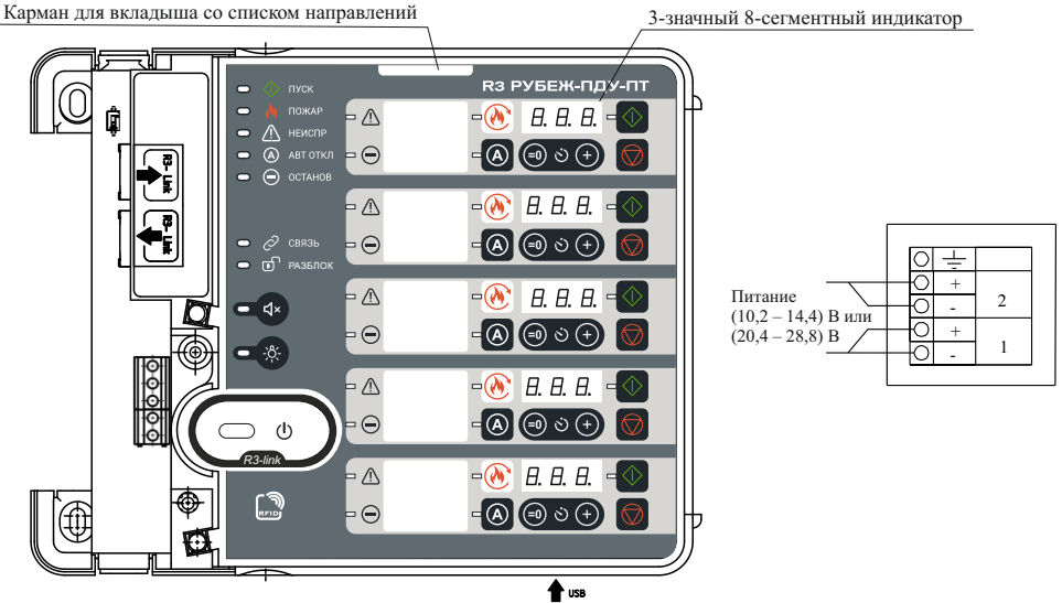
Рисунок 1 – Внешний вид и схема подключения прибора
