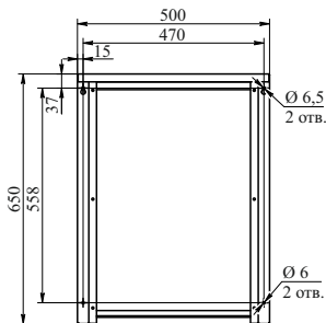
а) ШУ мощностью 45 кВт (IP31)
