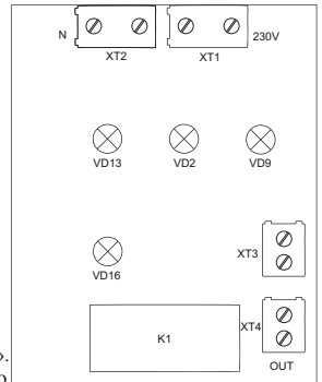
Рисунок 3 – Модуль контроля фаз
