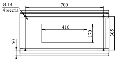
г) ШУ мощностью 250 кВт, вид снизу
