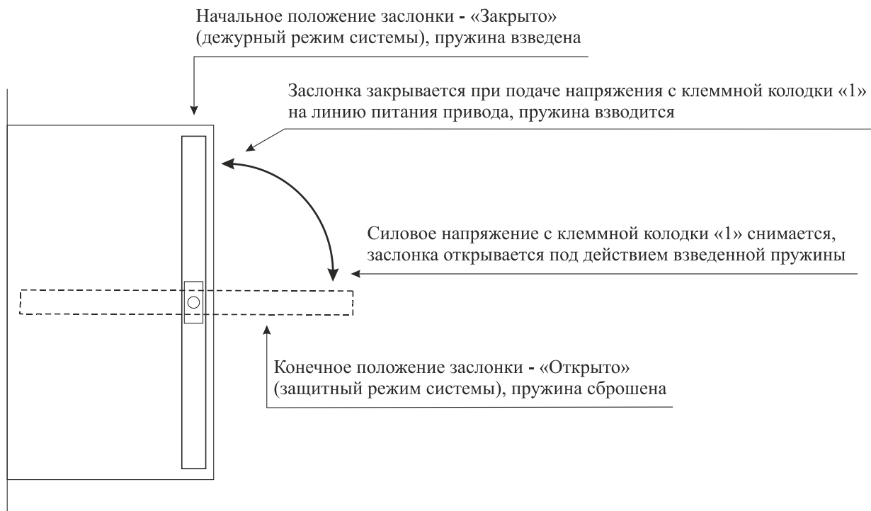
Рисунок 4.6 – Пример схемы реализации функции «Дымоудаление» для привода с возвратной пружиной
