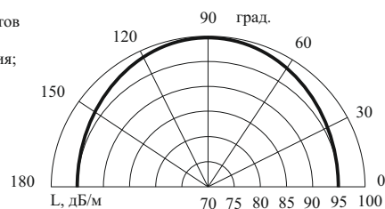
Рисунок 1 – Диаграмма направленности
