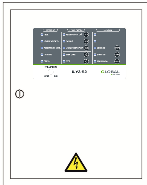
Рисунок 1 – Лицевая сторона ШУ
