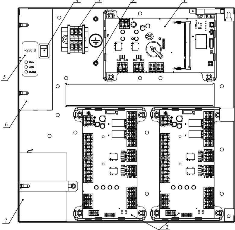
Рисунок 2 – Внутреннее устройство контроллера
