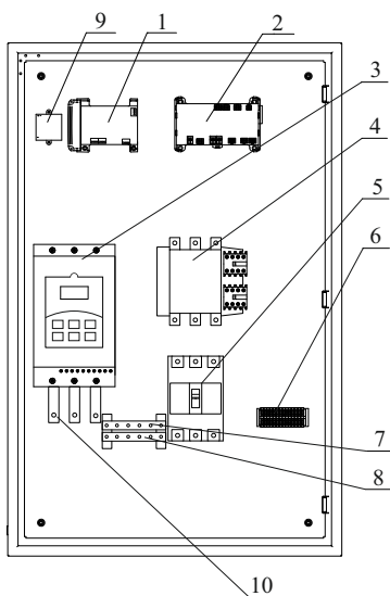
в) ШУ мощностью (55 – 75) кВт
