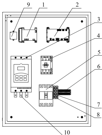
б) ШУ мощностью (30 – 45) кВт
