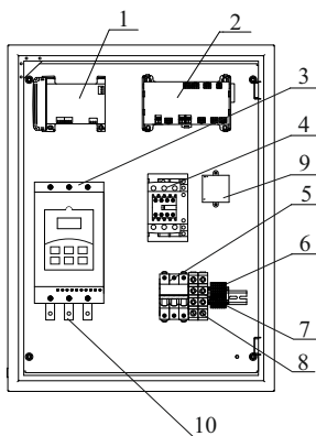
а) ШУ мощностью (1,5 – 22) кВт
