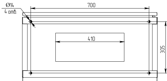
Рисунок 7 – Установочные размеры ШУ мощностью (90 – 250) кВт, вид снизу
