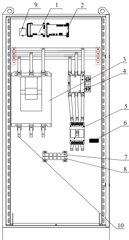
д) ШУ мощностью (90 – 250) кВт
