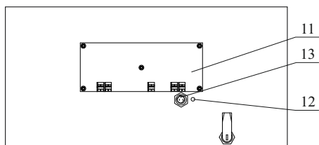
г) ШУ мощностью (1,5 – 250) кВт Вид на открытую дверь изнутри
