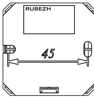
Рисунок 5 – Установочные размеры
