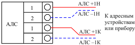
Рисунок 2 – Схема подключения
