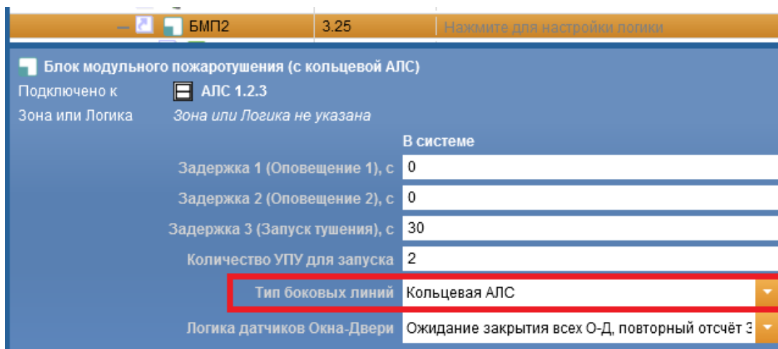
Рисунок 3.29 – Параметры БМП2
