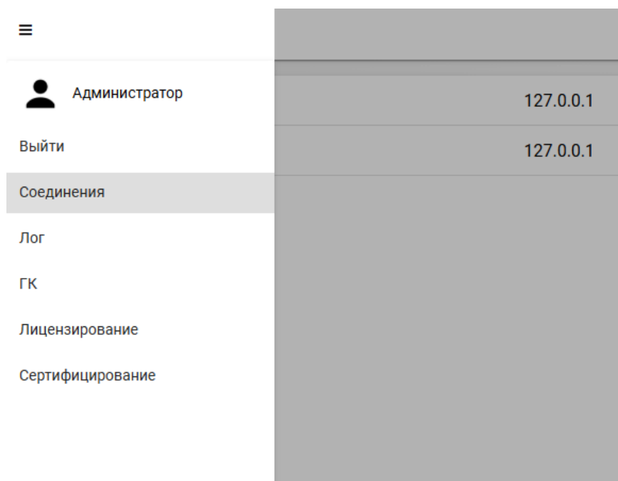
Рисунок 1.7 – Монитор сервера
