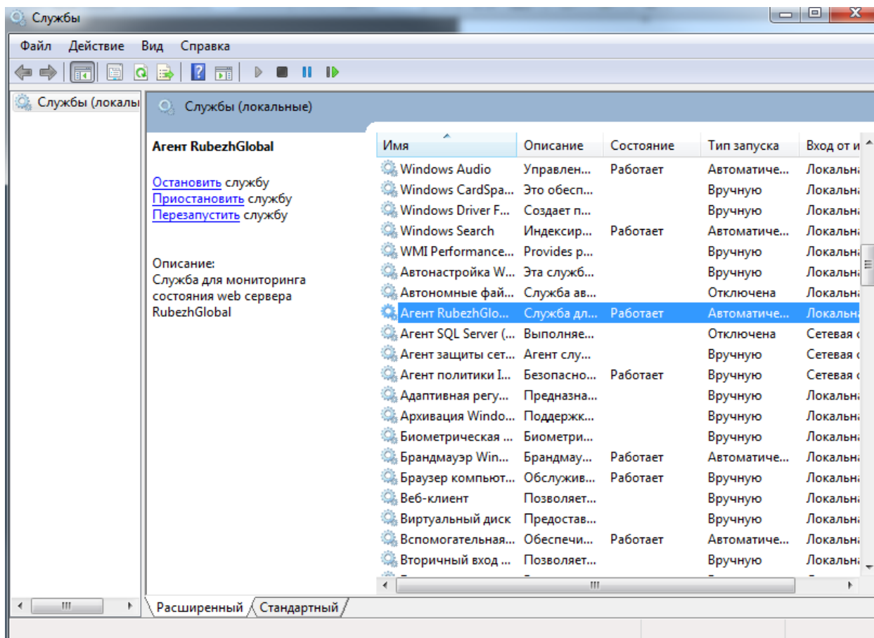
Рисунок 1.11 – Запуск службы
