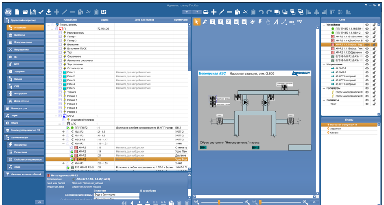
Рисунок 4.1 – Окно Планы
