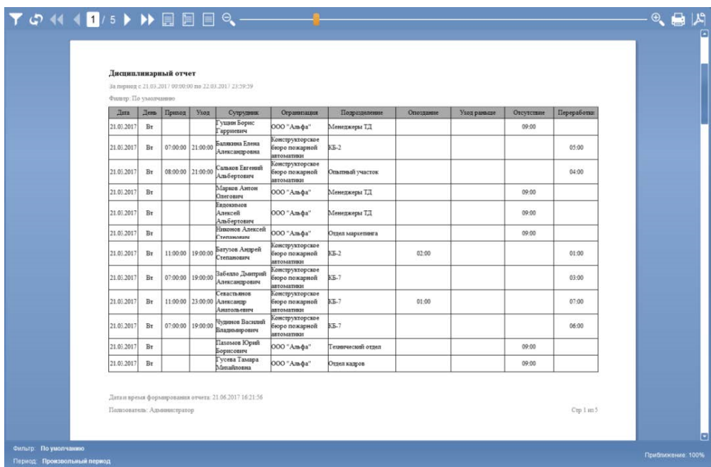
Рисунок 11.47 – Дисциплинарный Отчет
