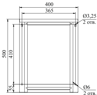
Рисунок 5 – Установочные размеры ШУ
