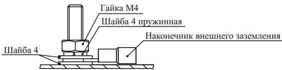
Рисунок 3 – Установка элемента заземления
