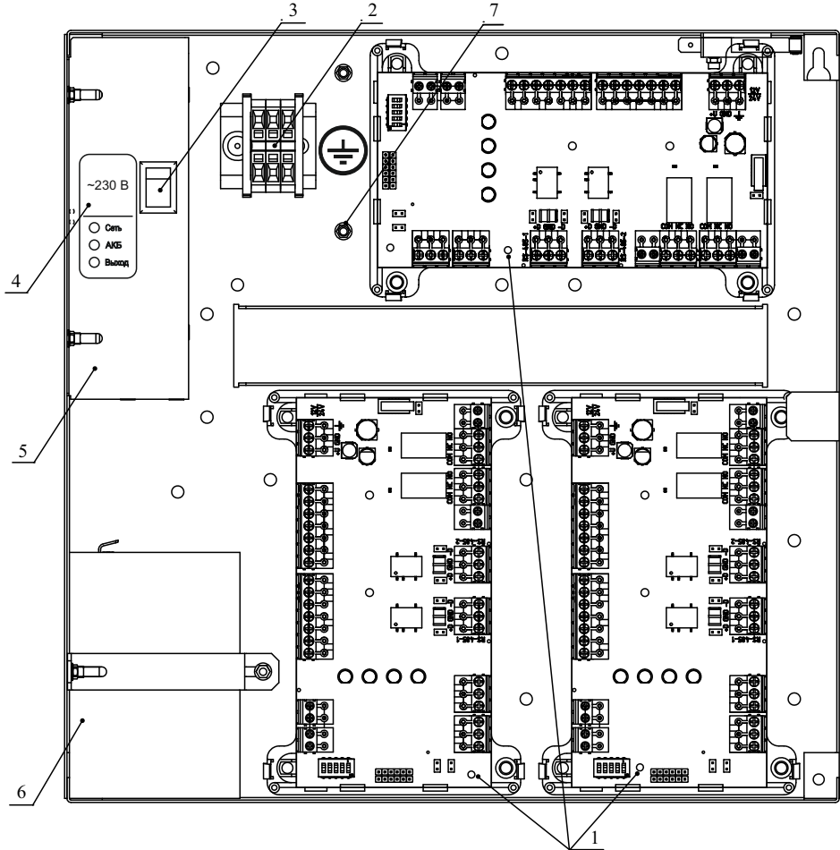
Рисунок 2 – Внутреннее устройство модуля
