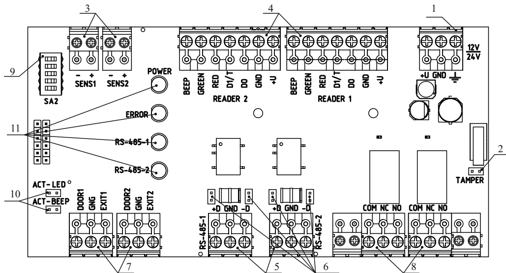
Рисунок 4 – Плата модуля
