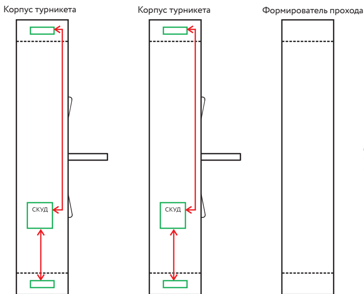
Рисунок 11.4 - Подключение без переноса считывателей в турникете 3V Model T/T(s) и формирователем прохода
