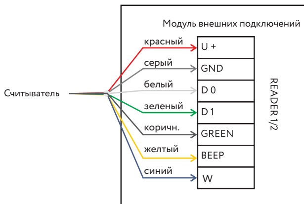
Рисунок 6.3 - Подключение считывателя к плате внешних подключений СКУД RUBEZH STRAZH
