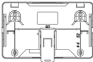
Рисунок 2 – Установочные размеры
