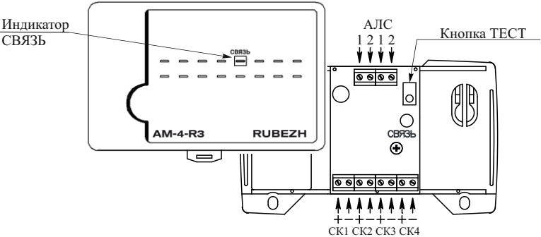
Рисунок 1 – Внешний вид крышки и основания с платой
