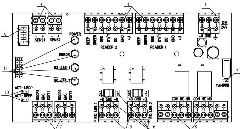
Рисунок 5 – Плата модуля внешних подключений контроллера
