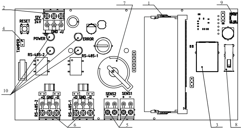
Рисунок 4 – Плата контроллера
