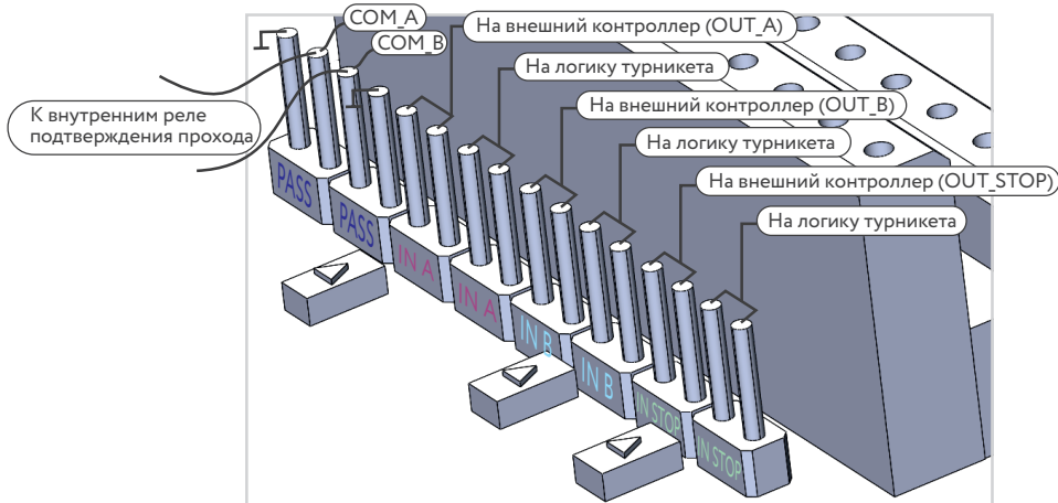
Рисунок 4.3 – Логическая схема использования джамперов пульта
