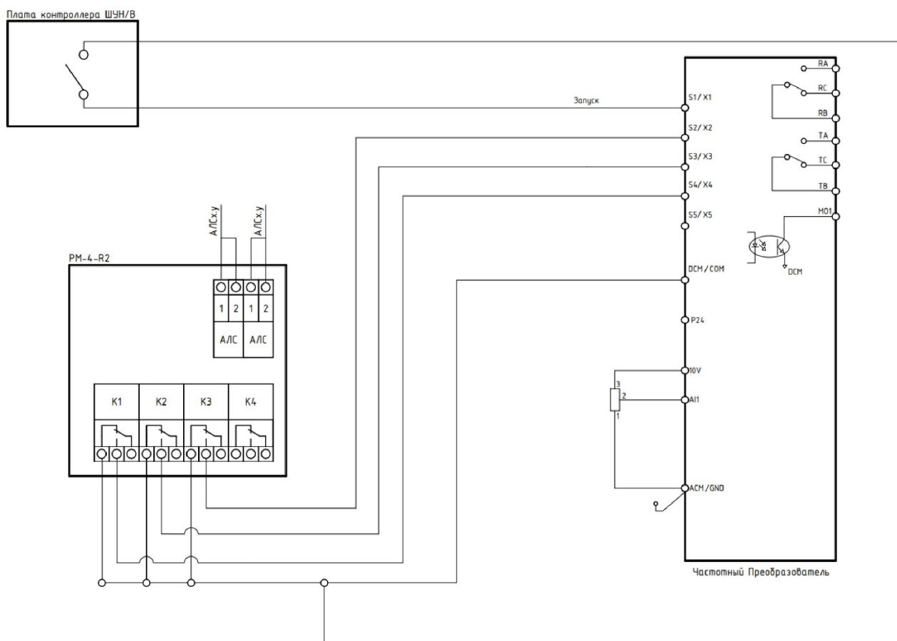
Схема подключения РМ-4-R2 и частотного преобразователя Instart.
