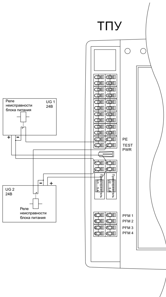
Рисунок 9 – Схема подключения с двумя источниками и выходом контроля неисправности блока питания типа «сухой контакт»
