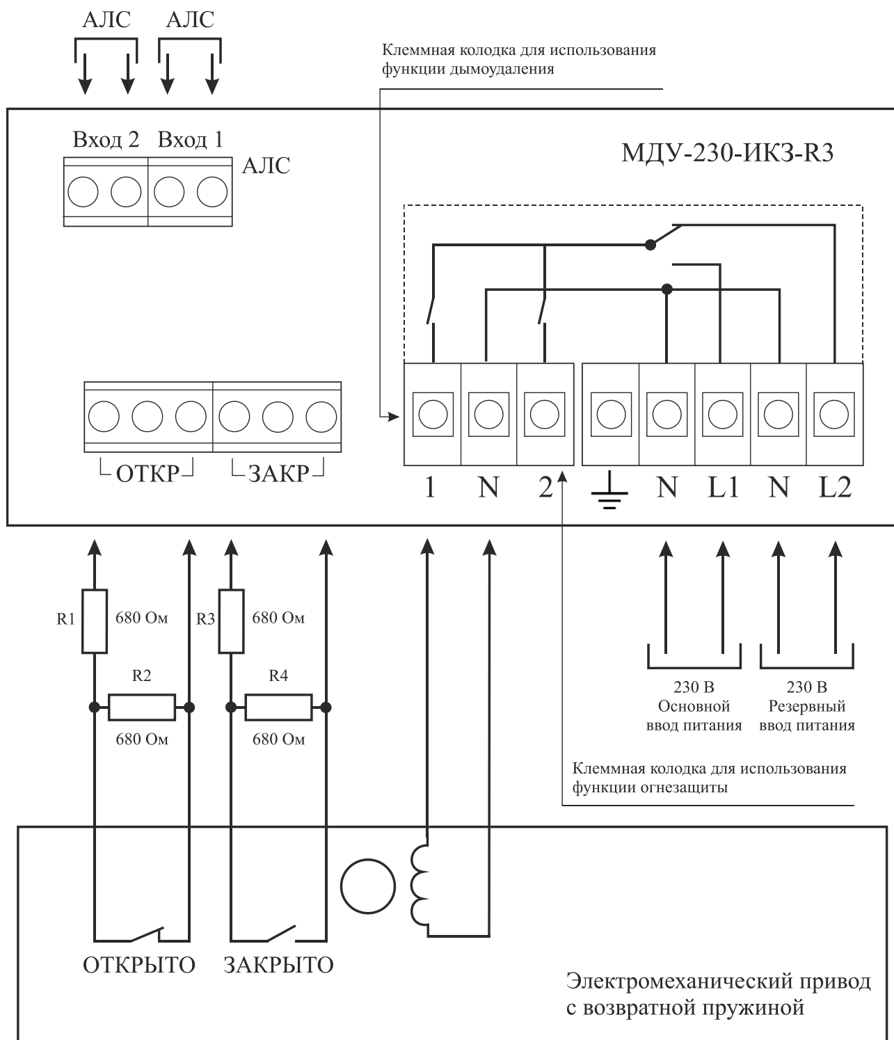
Рисунок 4.8 – Подключение привода с возвратной пружиной с номинальным напряжением 230 В для выполнения функции дымоудаления (контакты, коммутирующие напряжение, изображены в положении, соответствующем обесточенному состоянию МДУ)
