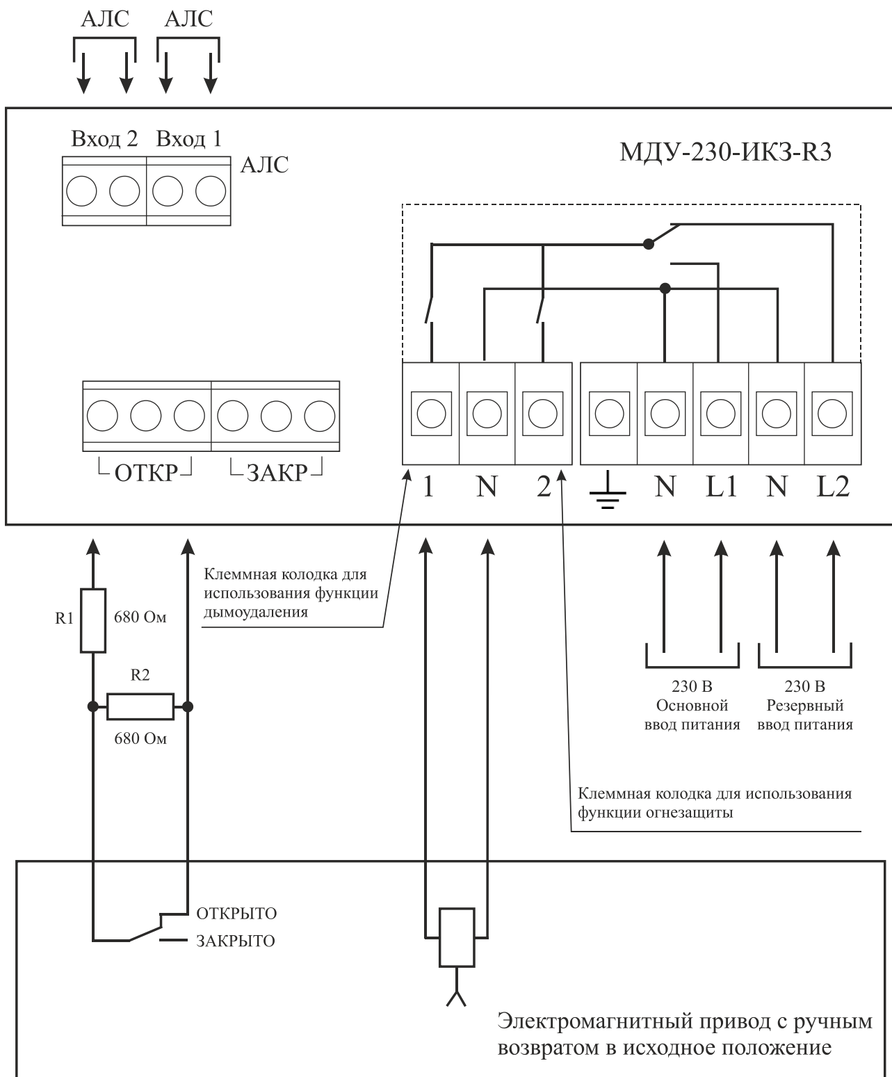
Рисунок 4.10 – Подключение электромагнитного привода с ручным возвратом в исходное положение с напряжением 230 В для функции дымоудаления (контакты, коммутирующие напряжение, изображены в положении, соответствующем обесточенному состоянию МДУ)
