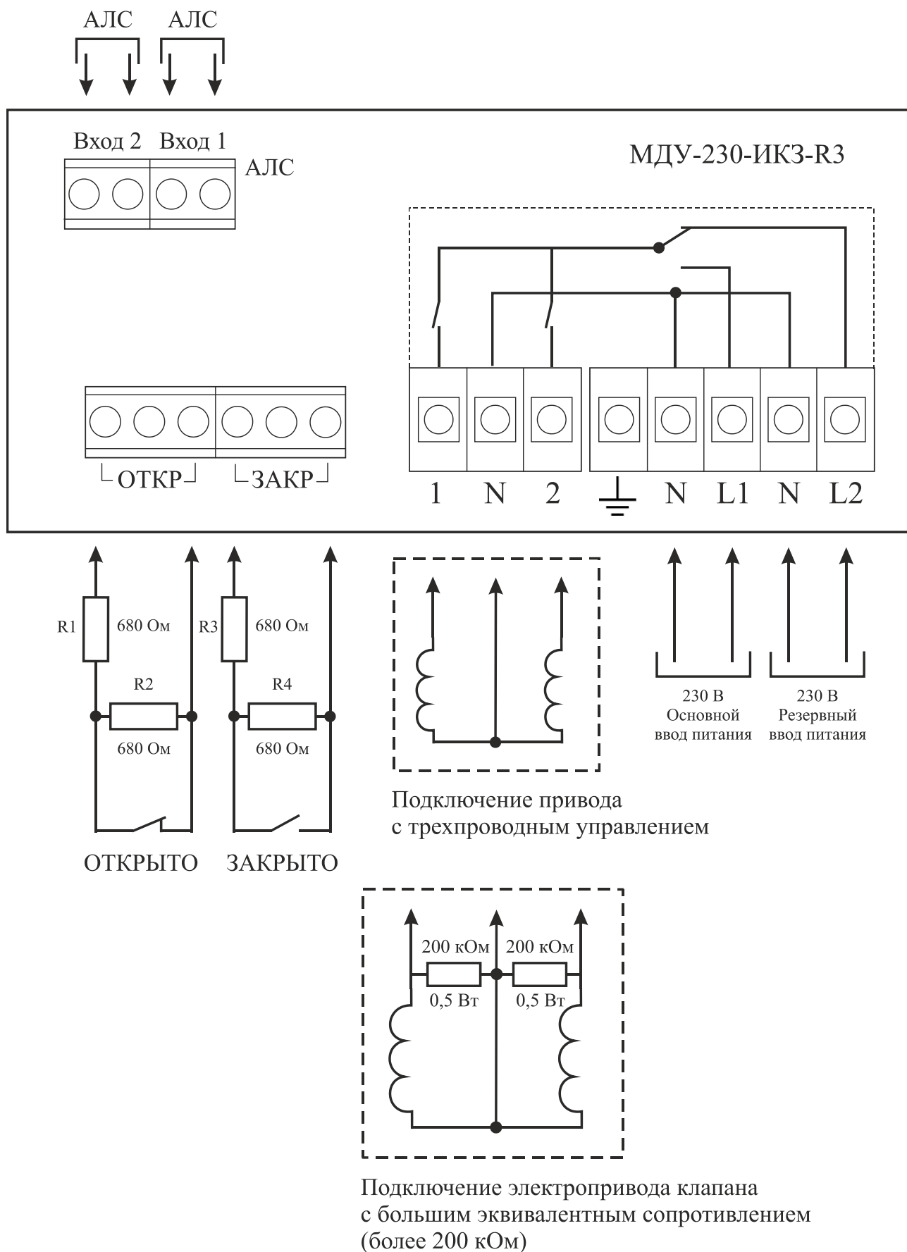
Рисунок 4.4 – Подключение реверсивного привода с концевыми выключателями с номинальным напряжением 230 В (контакты, коммутирующие напряжение, изображены в положении, соответствующем обесточенному состоянию МДУ)
